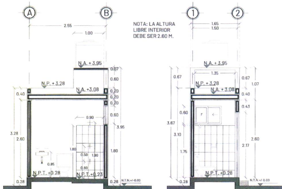
CORTE X-X'
