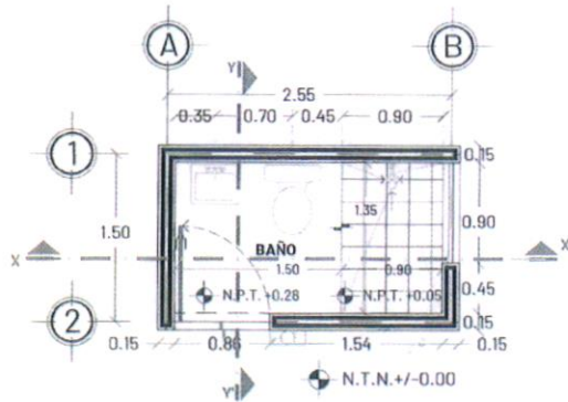
PLANTA ARQUITECTÓNICA
