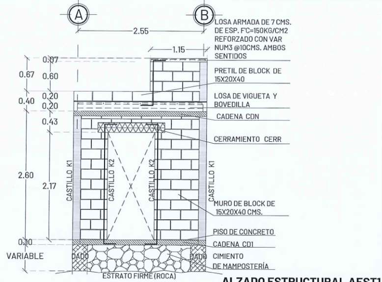
ALZADO ESTRUCTURAL AEST1
