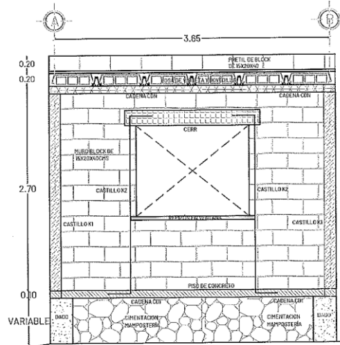
ALZADO ESTRUCTURAL AEST2
