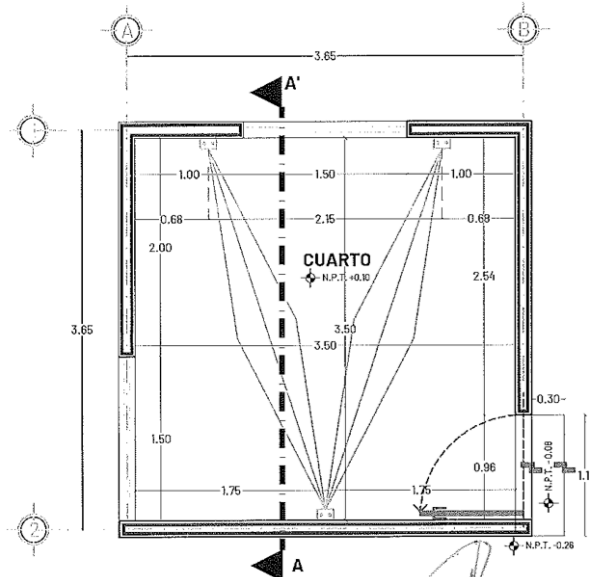
PLANTA ARQUITECTÓNICA
