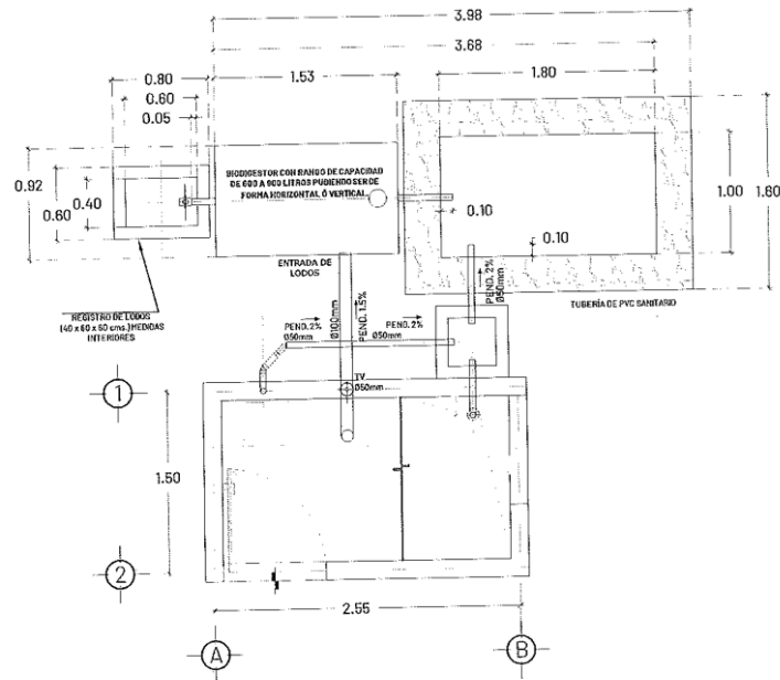
PLANTA DE INSTALACIÓN SANITARIA
