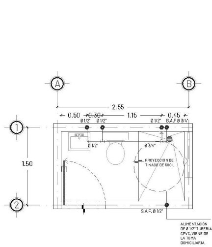
PLANTA DE INSTALACIÓN HIDRÁULICA
