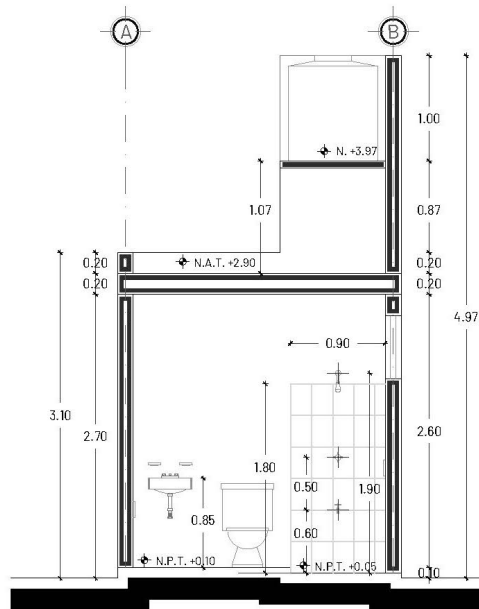
CORTE X-X'
