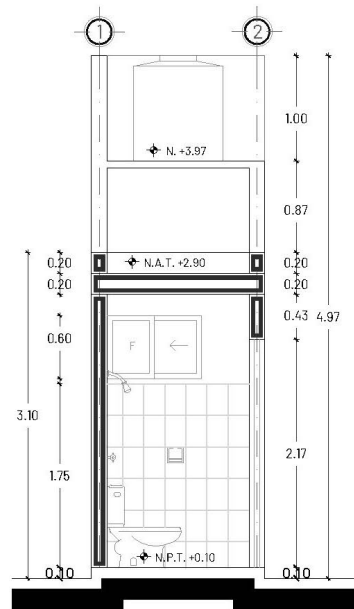
CORTE Y-Y'
